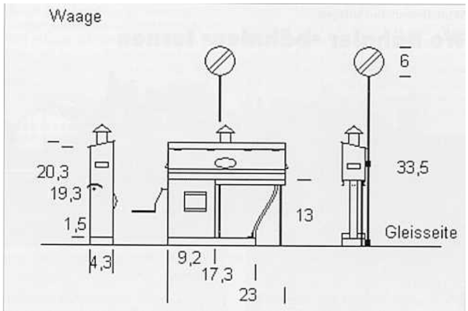
Plan der Gleiswaage mit den genauen Massangaben (Zeichnung: H. Berneth)
