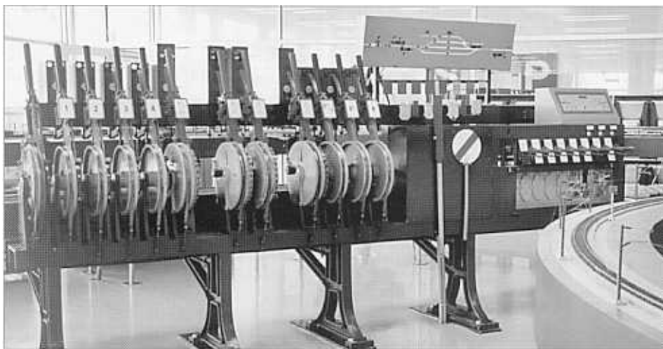
Ein Schmuckstück: Das mechanische Stellwerk von Hirtfelden ist funktionstüchtig. (Foto: D. Felix)
