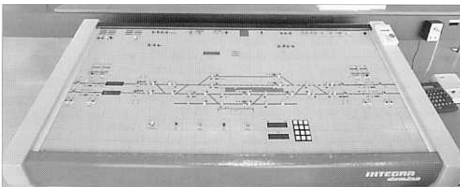
Aus der Sicht des Fahrdienstleiters: Das Domino-55-Stellwerk von Dachsburg mit dem dazugehörigen Modellbahnhof (Foto: D. Felix)
