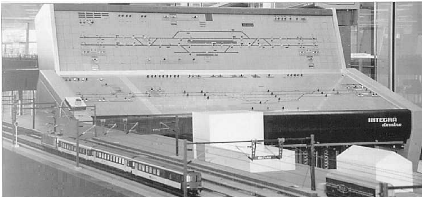
Vorbild und Modell: Der Modellbahnhof Fusio mit dem original grossen Domino-69-Stellwerk (Foto: D. Felix)
