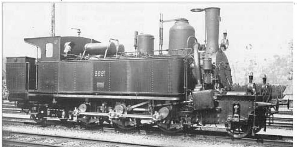
Schnellzug-Tenderlokomotive Eb 3/5, genannt «Salondampfer» (Foto: VHS)
