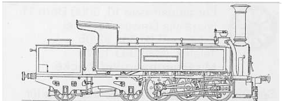
Güterzug-Tenderlokomotive System Engerth Ed 3/5 (Skizze: A. Moser, Dampftrieb der Schweizerischen Eisenbahnen)
