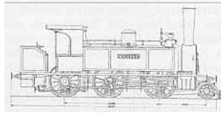
Personenzuglokomotive Eb 3/4 nach Umbau (Skizze: Verlag Eisenbahn)
