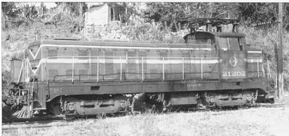
Elektrifizierte 040-DE der kubanischen Staatsbahn in Sibacoá (17.2.1998; P. Willen)
