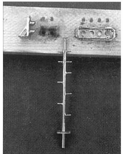
Lötlehre für die Tafeln, Tafeln mit Gerüst verlötet
