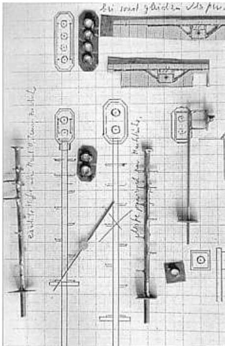
Teile der Modellmaste, oben noch nicht ausgeschnittene Gerüste für die Signaltafeln, zweite (zu grosse) Signalzeichnung von links: basierend auf dem Mastdurchmesser von 1,5 mm
