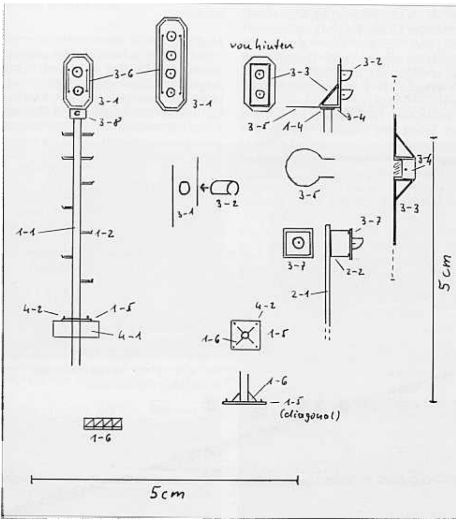
Bauzeichnung für ein Hauptsignal und ein Blinklicht
