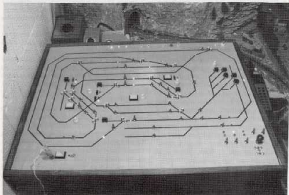
Bild 2: Überblick über ein Gleisbildstellwerk (Foto M. Klausner)
