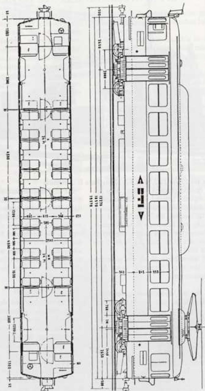
Typenskizze der BTI-Fahrzeuge
