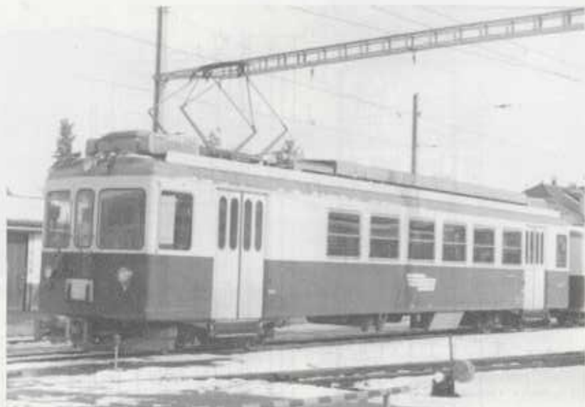
Der LEB-Be 4/4 27 am 21.2.93 in Echallens (Foto E. Jordanis)
