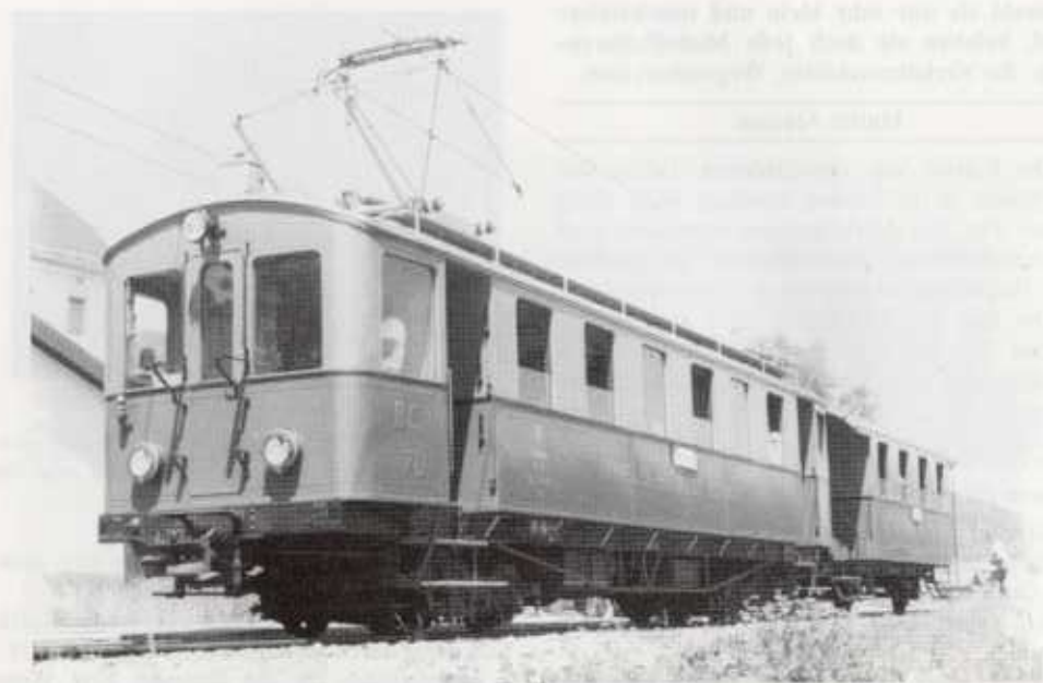
Der BCe 2/4 70 im Einsatz als Nostalgiezug (Les Ponts de Martel, 21.7.91; Foto E. Jordanis)
