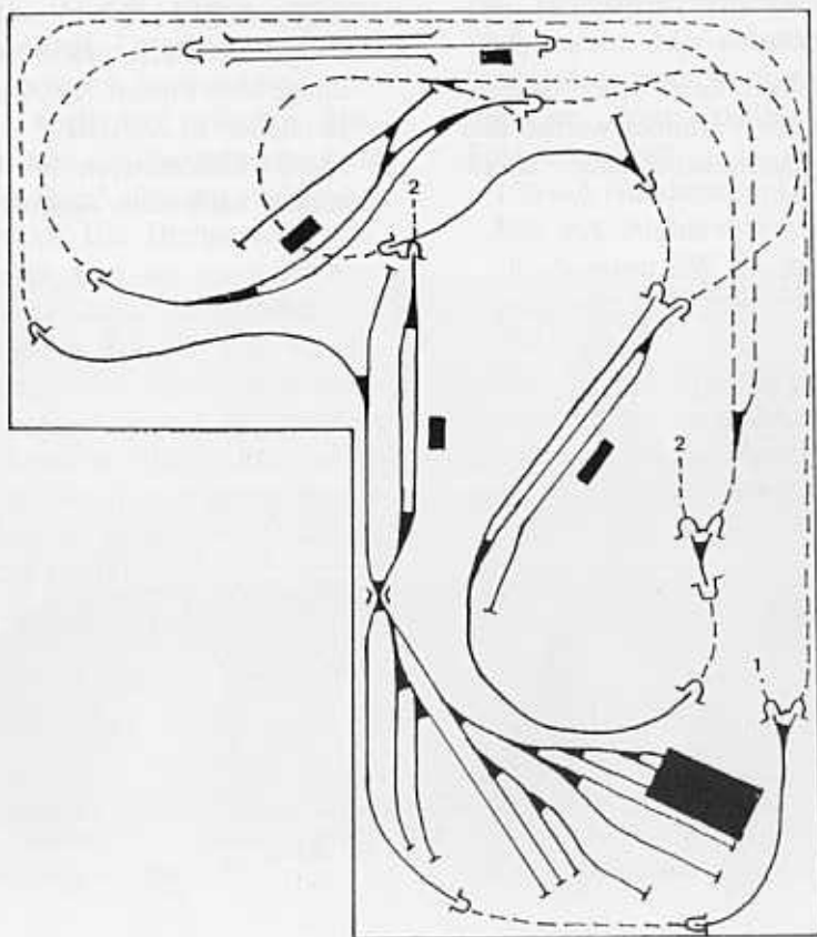
Übersichtsskizze
