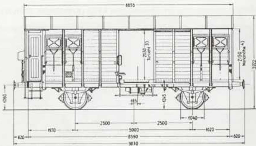
Typenskizze K3 mit Bremserhaus
